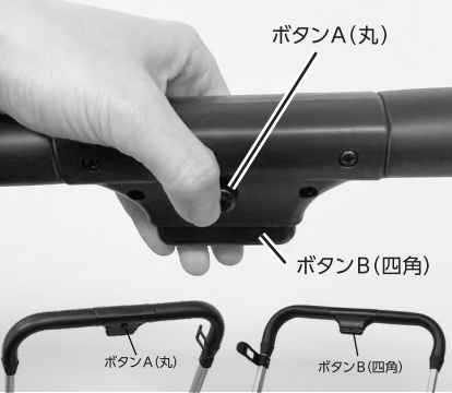
③ハンドルの内側にあるボタンAを親指で押しながら、ボタンBを強く押すように握ります。 ④ボタンBを押したままハンドルを前方に押し倒してフレームをたたみます。
