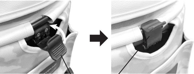
フードカバー固定用バックル
